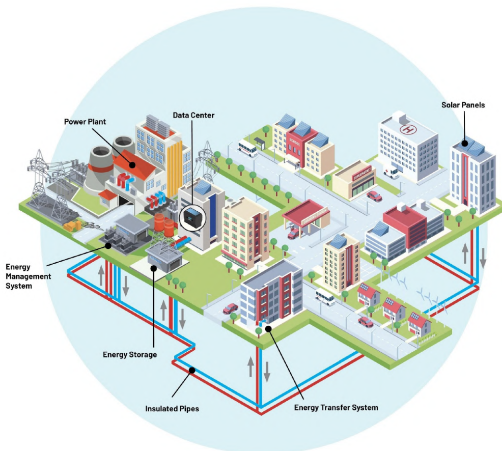
Figura1. Schema di un impianto di recupero e stoccaggio del calore scaricato da un Data Center integrato nel sistema energetico della città.
